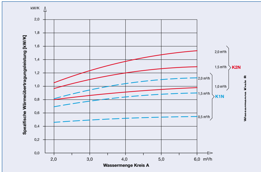
Spezifische Wärmeübertragungsleistung [kW/K] K1N und K2N
