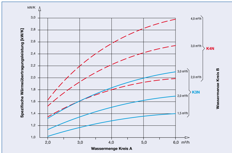
Spezifische Wärmeübertragungsleistung [kW/K] K3N und K4N
